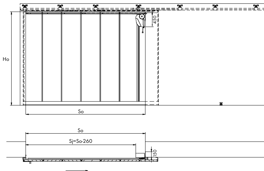
Napęd w bramie jednoskrzydłowej - widok wewnątrz
